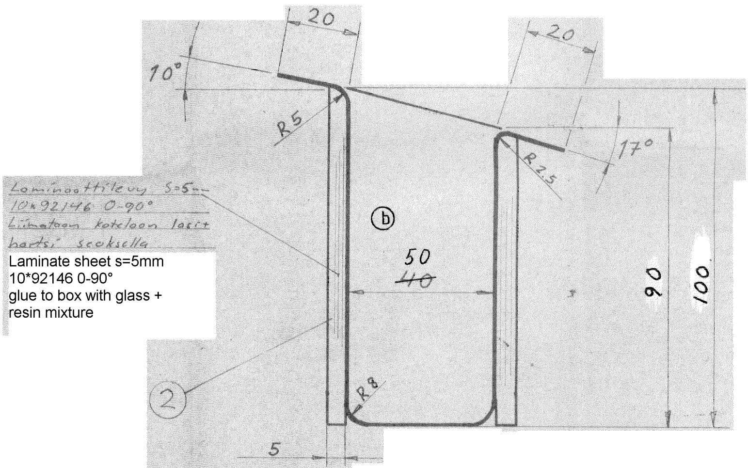
Leikk. A-A Cut A-A
