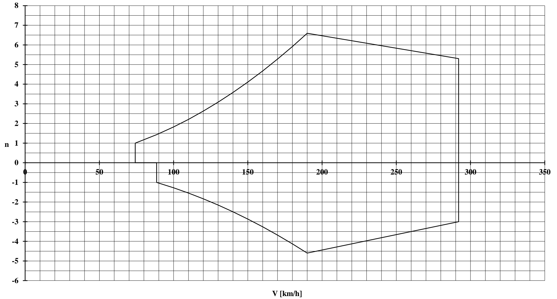
PIK-20TurboD. Liikehtimisen (V,n)-piirros taitolentoluokassa (OSTIV 1971 Acrobatic). m = 360 kg
