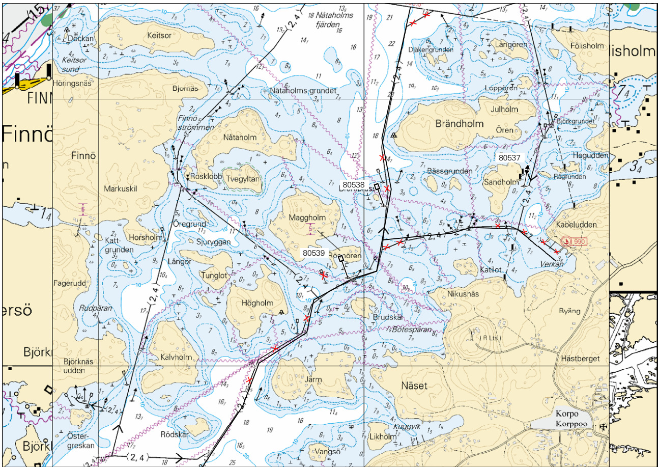
Ei merikartan mitttakaavassa - Inte i sjökortets skala - Not to scale of chart
