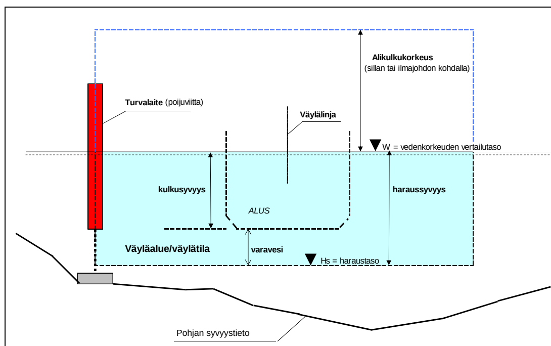
Kuva 1. Väyläpoikkileikkaus, periaatepiirros (Liikennevirasto: Vesiväyliin liittyviä käsitteitä, Dnro 1342/610/2005, 31.10.2011)
