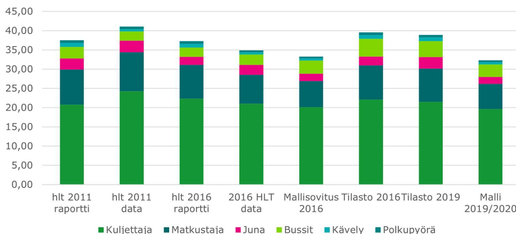
Kuva 103. Suoritteet per henkilö 2010-luvun tilastoissa, henkilöliikennetutkimusraporteissa (hlt) ja niiden aineistoissa sekä niiden pohjalta sovitetussa yksilömallissa.
