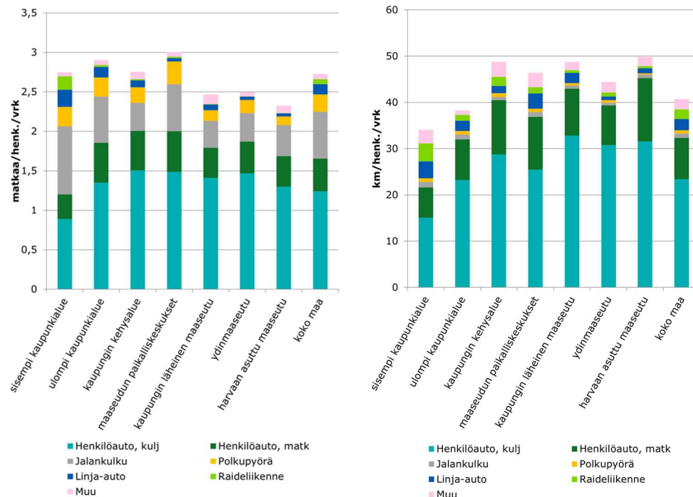
Kuva 15. Päivittäinen matkamäärä ja liikennesuorite kulkumuodoittain erityyppisillä alueilla (HLT 2016).
