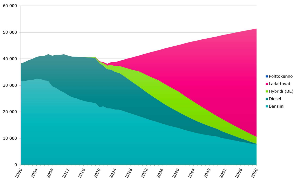
Kuva 34. Henkilöautojen ajoneuvosuoritteet käyttövoimittain 2000 - 2021 ja ennuste 2022 - 2060.
