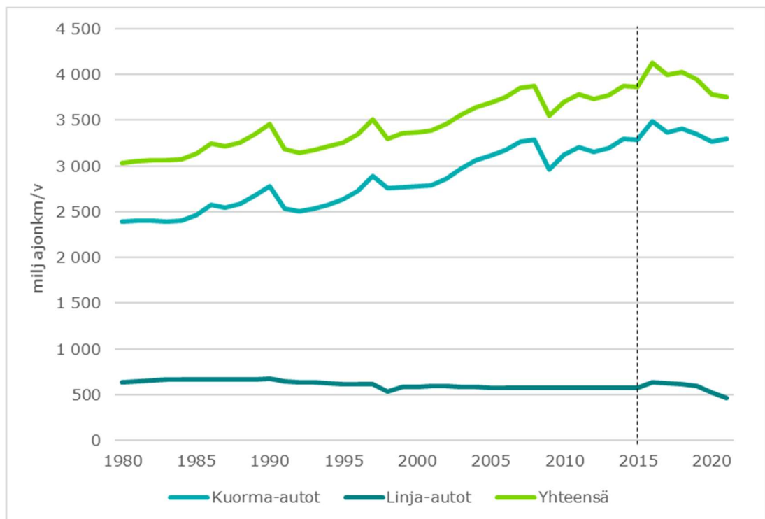
Kuva 46. Kuorma- ja linja-autojen suoritteiden toteutunut kehitys 1980 - 2021. Tilastointitavan muutoksen vuoksi vuoden 2015 jälkeen luvut eivät ole täysin vertailukelpoisia aiempien vuosien kanssa.
