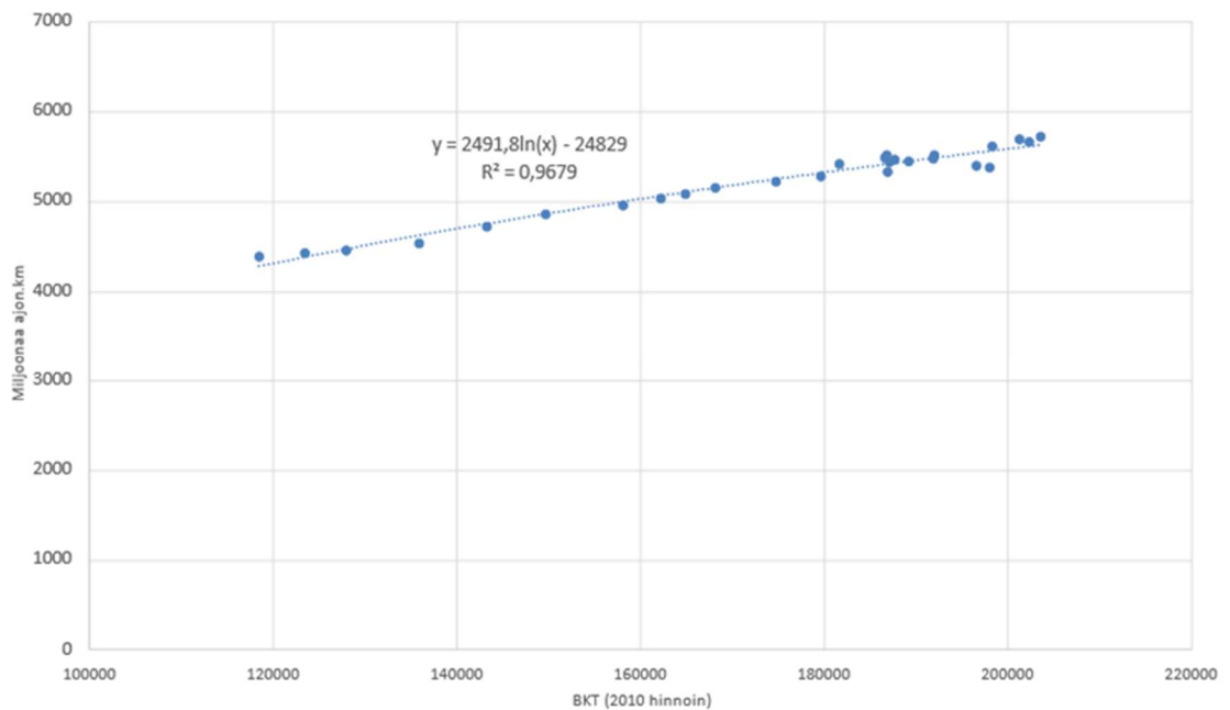
Kuva 5. Pakettiautoliikenteen ajosuorituksen ja BKT:n välinen suhde vuosina 1994-2020.
