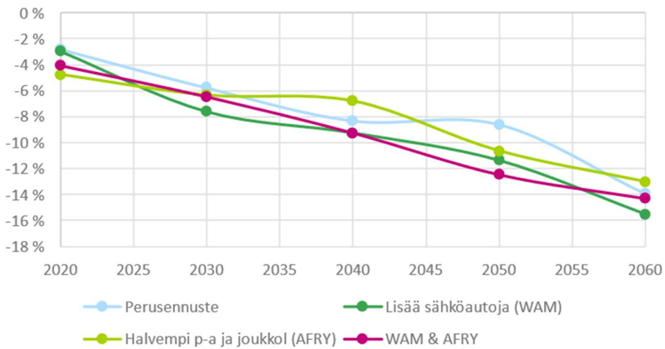
Kuva 123. Linja-autoliikenteen suoritteiden muutos eri herkkyystarkasteluissa.
