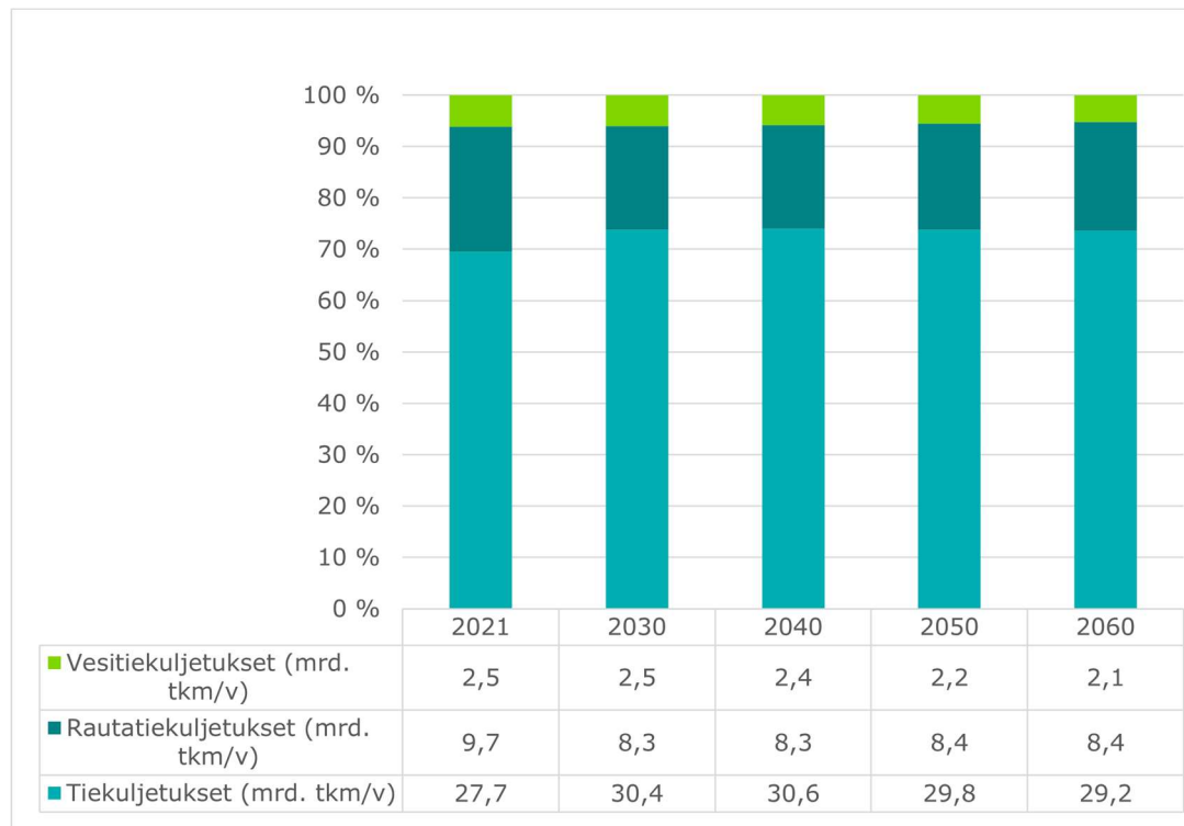
Kuva 44. Kotimaan tavaraliikenteen ennustettu kehitys kuljetustavoittain.
