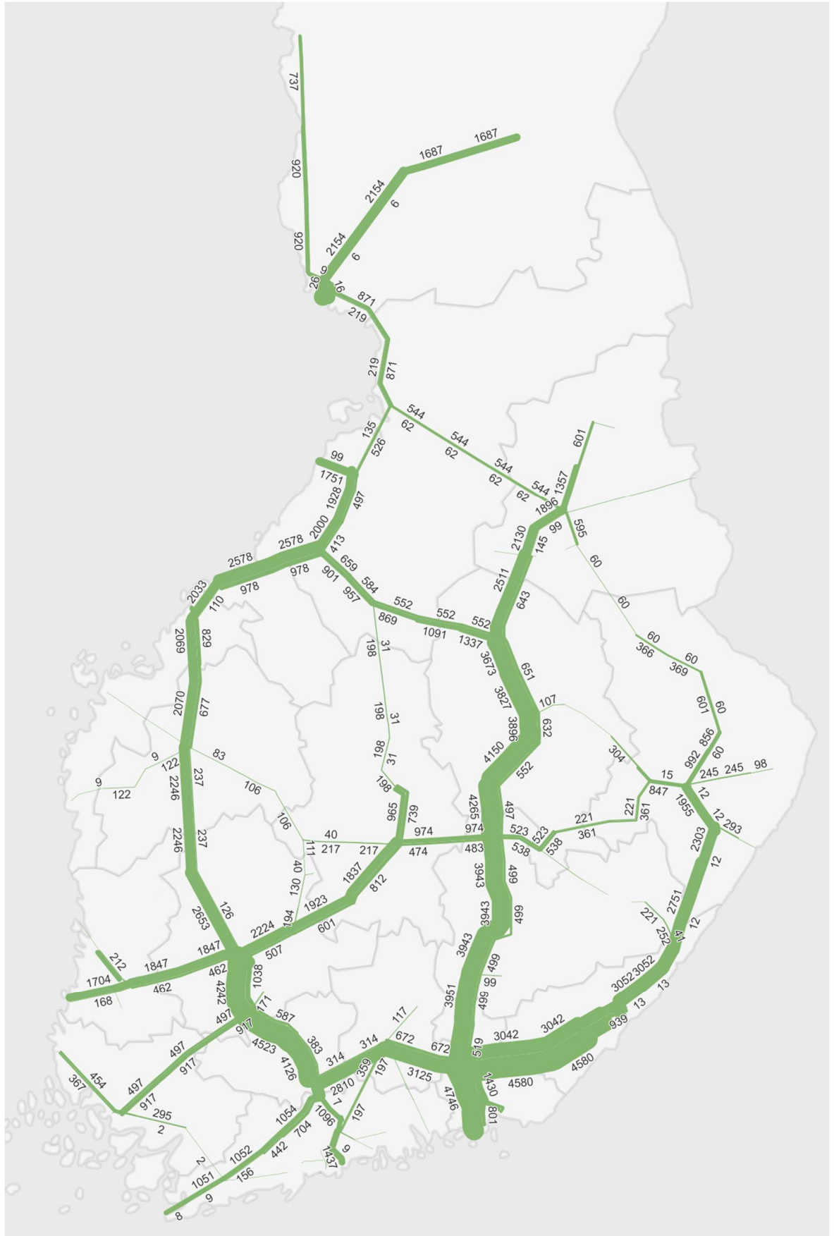
Kuva 73. Vuoden 2060 ennustetut kuljetusmäärät rataverkolla (1 000 nettotonnia).
