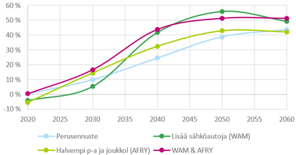
Kuva 122. Raideliikenteen suoritteiden muutos eri herkkyystarkasteluissa.
