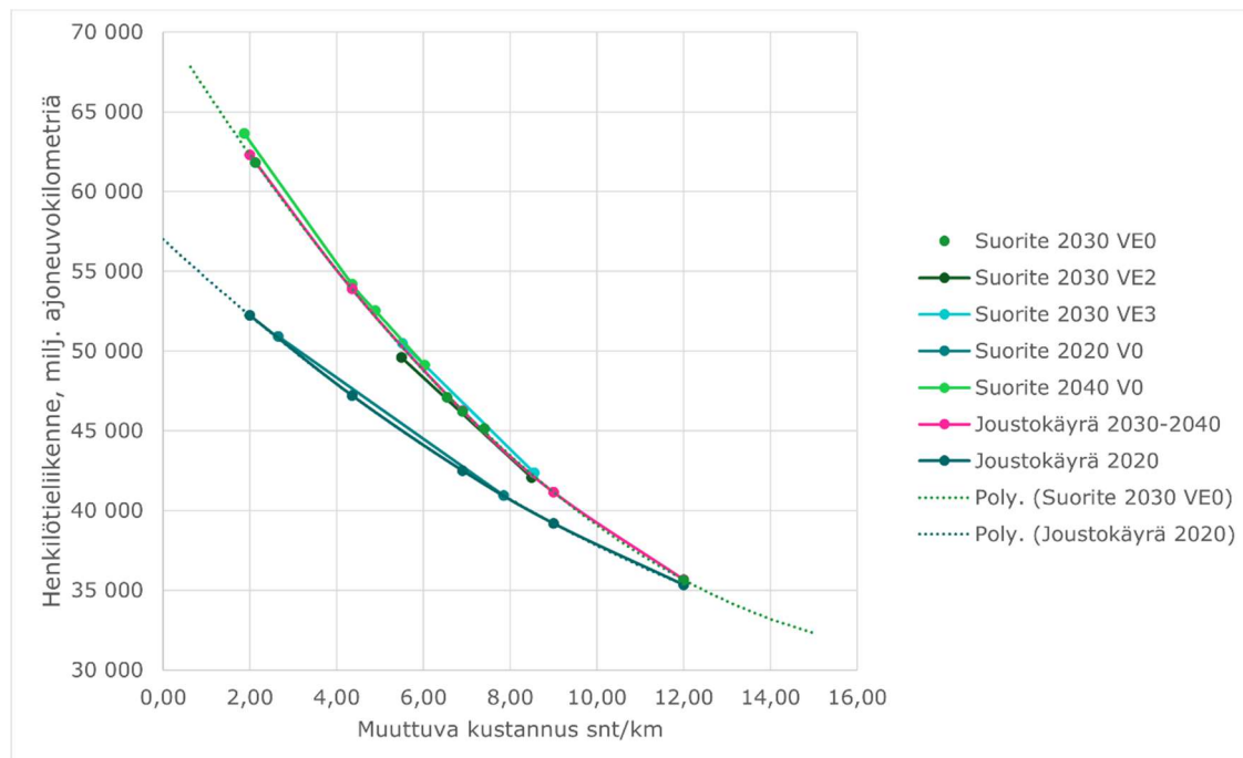
Kuva 105. Autoilun muuttuvan ajokustannuksen ja suoritteiden välinen suhde tieliikenteen päivitettyissä ennusteissa vuonna 2021.
