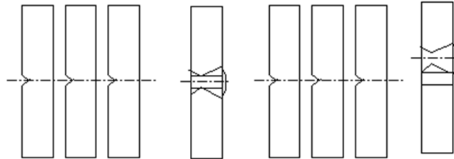
Hitsausliitoksen keskikohta
