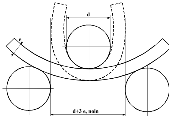
Taivutuskokeen kaaviokuva
