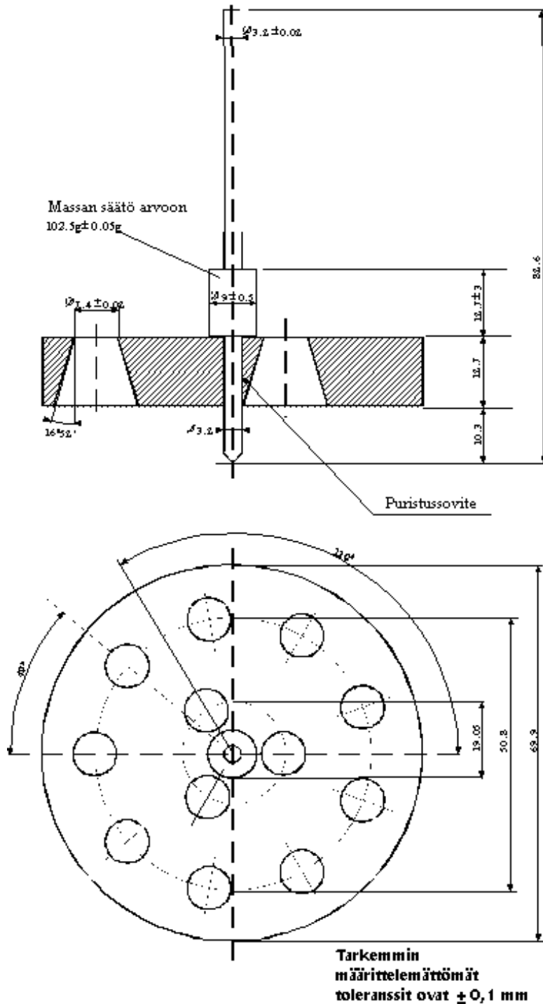
Kuva 1: Penetrometri
