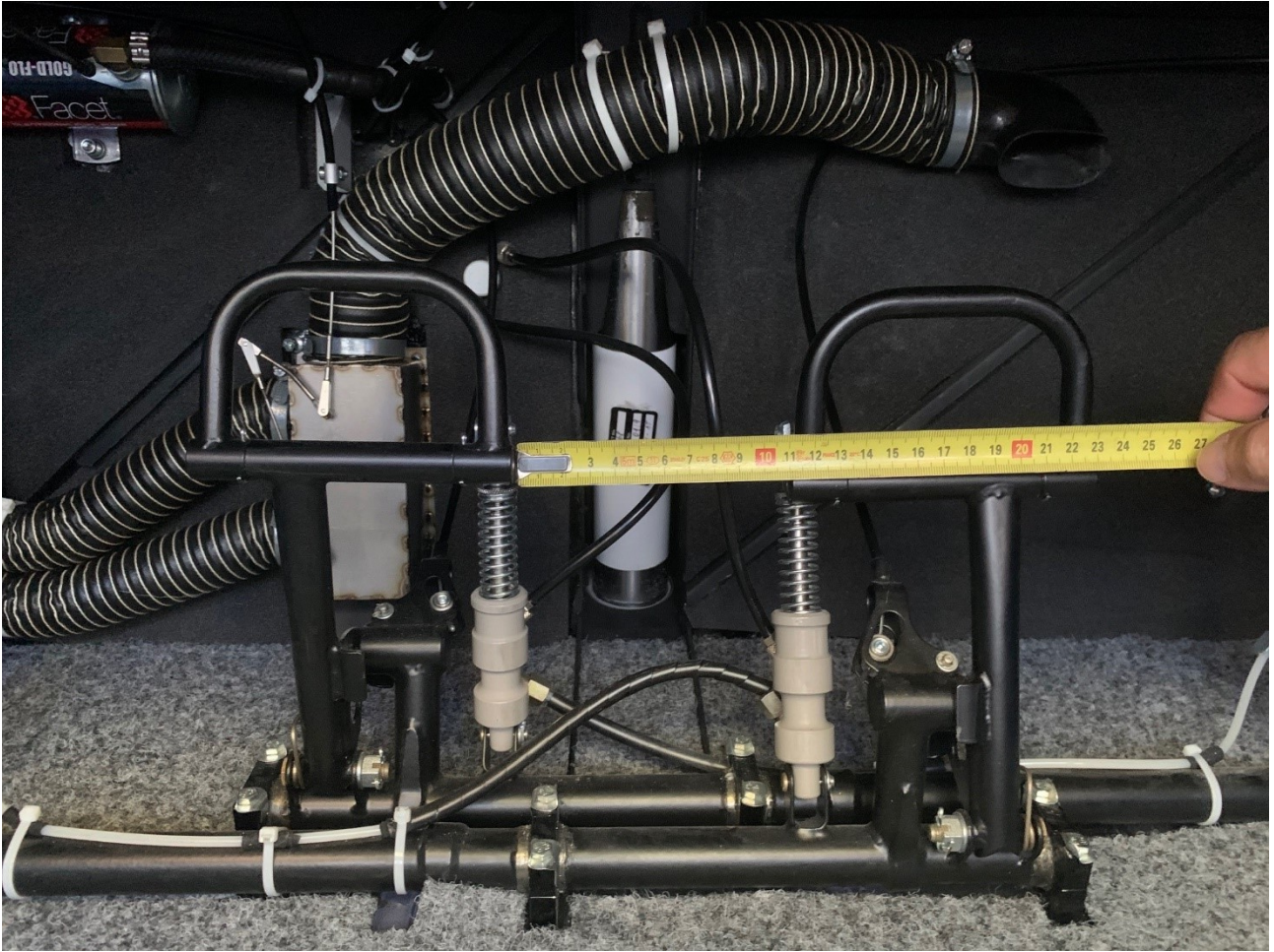
Kuva 2. Eurostar SLW -mallin poljinjärjestely, oikean- ja vasemmanpuoleisen ohjaajan poljinten välinen etäisyys.
