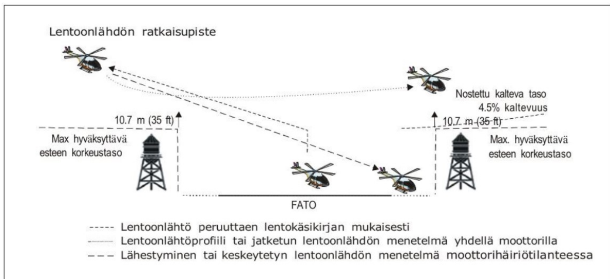
Kuva 4-4. Esimerkki nostetusta kaltevasta tasosta operaatioille suorituskykyluokassa 1
