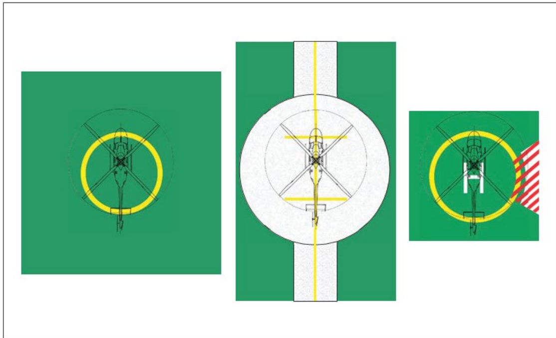
Kuva 5-8. Kosketuskohtamerkintöjä. (Vasemmalla) Monisuuntainen TDPC ilman rajoituksia. (Keskellä) yksisuuntainen merkintä keskilinjamerkinnän kanssa. (Oikealla) Monisuuntainen TDPC, jossa kielletyn laskeutumissektorin merkintä
