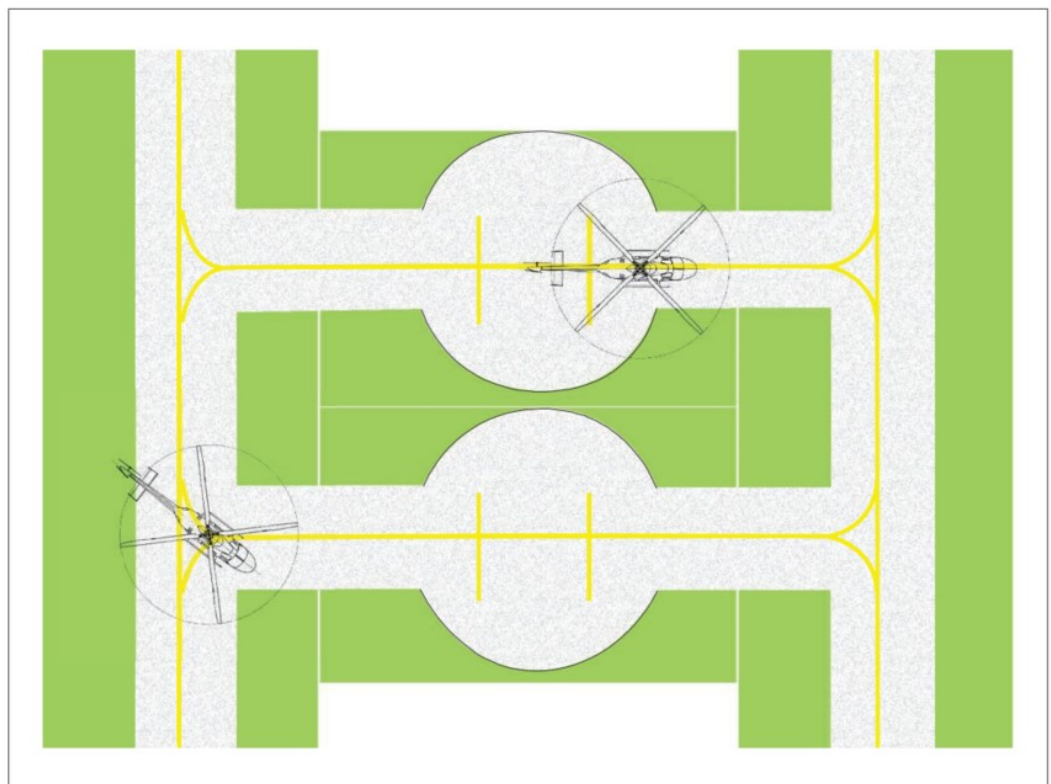
Kuva 3-6. Seisontapaikat; samanaikainen käyttö sekä läpikulutus (maarullaus: rullausreitti/maarullausreitti)
