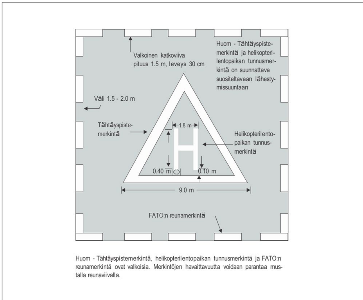
Kuva 5-1. Yhdistetty helikopterilentopaikan tunnus, tähtäyspistemerkintä ja FATO:n reunamerkintä. Kuva ei ole mittakaavassa.
