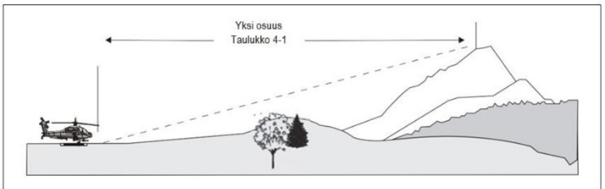
c) Lähestymis- ja lentoonlähöpinta - "C" kaltevuuskategoria - arvo 12.5%
