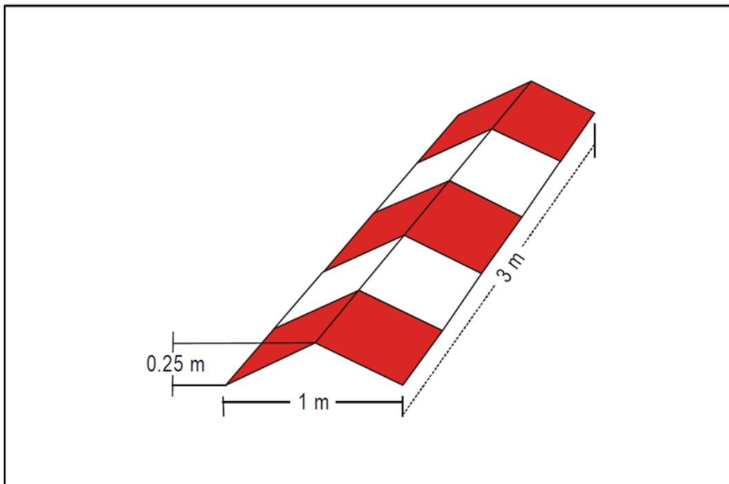
Kuva 5-6. Kiitotietyypisen FATO:n ulkoreunan reunamerkki
