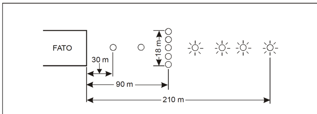
Kuva 5-13. Lähestymisvalojärjestelmä
