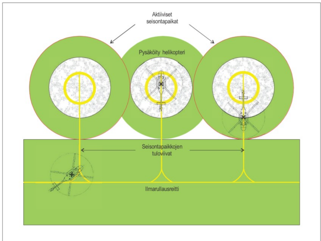
Kuva 3-8. Seisontapaikat kääntymiselle sekä ei-samanaikaiselle käytölle ja ilmarullausreitti – uloimmat seisontapaikat aktiivisia
