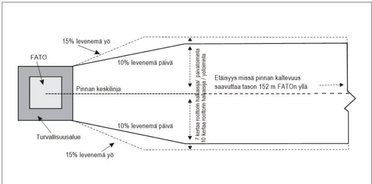
Kuva 4-2. Lähestymis- /lentoalähtöpinnan leveys
