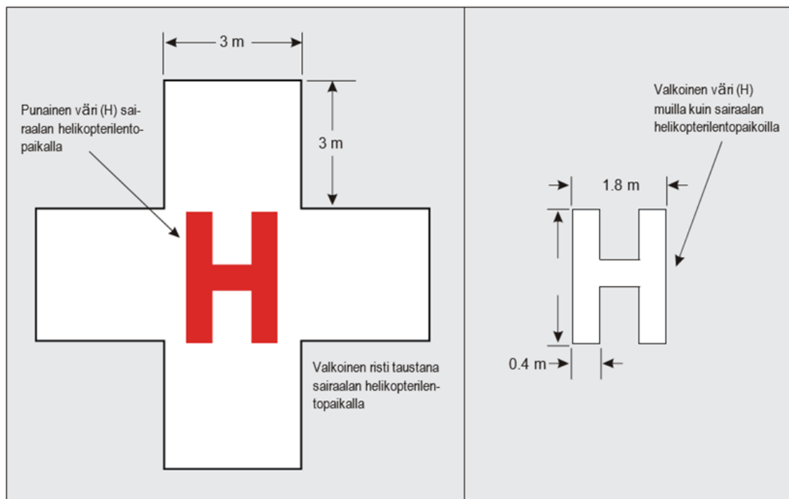
Kuva 5-4. Sairaalan helikopterilentopaikan tunnusmerkintä (vasemmalla) ja helikopterilentopaikan tunnusmerkintä, muut kuin sairaalan helikopterilentopaikat (oikealla).
