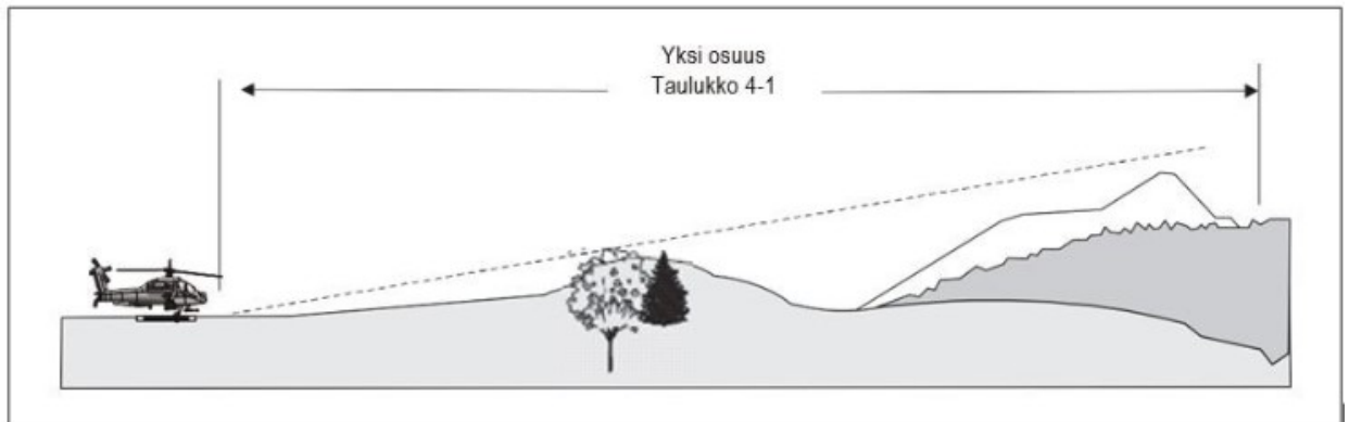
a) Lähestymis- ja lentoonlähöpinta - "A" kaltevuuskategoria - arvo 4.5%
