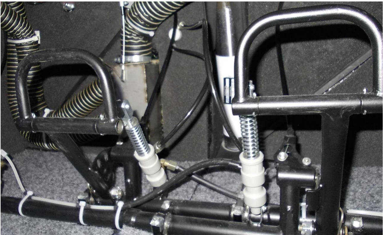
Model Eurostar SLW 600kg
